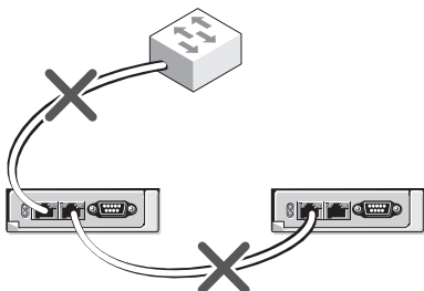
図 2-4. CMC ネットワーク接続の正しくないケーブル接続 – CMC が 2 つ
